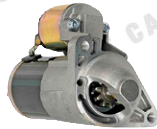
SM-2815 1.4kw,CW,11T,PMGR
