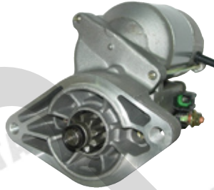
SN-1700 1.4kw,CW,9T
