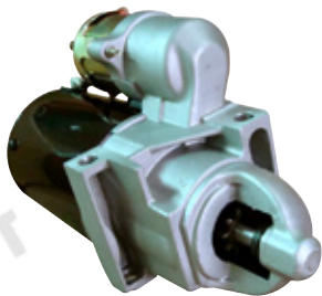
SD-1470 1.6kw,CW,9T,SD260
