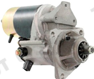
SN-0856 4.5kw,CW,11T
