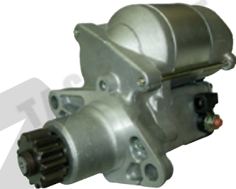
SN-1404 1.4kw,CCW,13T
