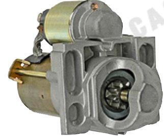
SD-2336 1.1kw,CW,9T,PG260D
