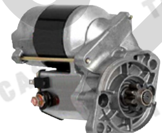
SN-2103 1.4kw,CW,9T
