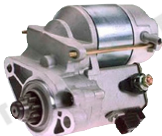
SN-1709 1.4kw,CW,9T
