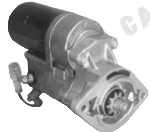
SN-1046 2.0kw,CW,9T
