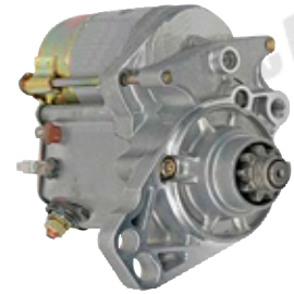
SN-1008 1.0kw,CW,9T
