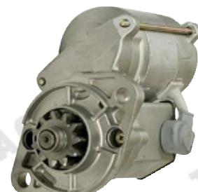
SN-8197 1.4kw,CW,11T
