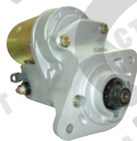
SN-8196R 1.4kw,CW,9T
