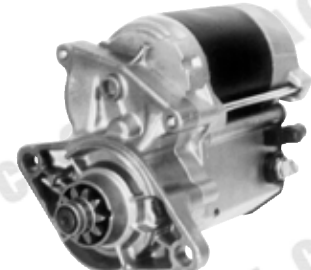
SN-1219 1.4kw,CCW,10T
