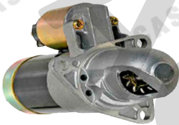
SM-1773 1.7kw,CCW,12T,PMGR
