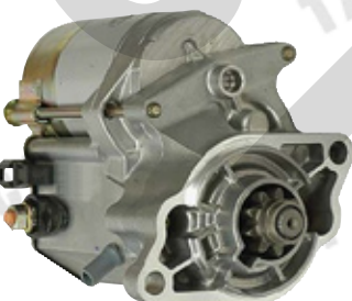
SN-8322 1.2kw,CW,9T
