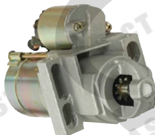
SD-1474 1.4kw,CW,11T,PG260L
