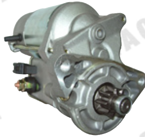
SN-1699 1.8kw,CW,9T
