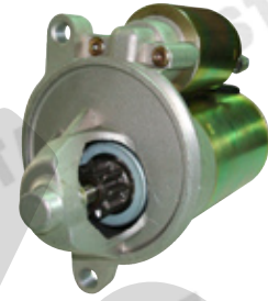
SF-1885 1.4kw,CW,10T,PMGR
