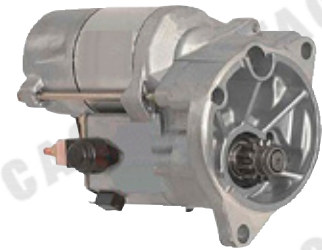
SN-2072 1.8kw,CW,11T
