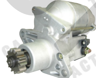
SN-14041 1.4kw,CCW,13T
