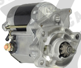
SN-0982 1.4kw,CW,9T
