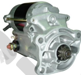
SN-2055 1.4kw,CW,9T
