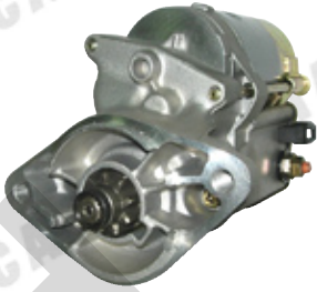
SN-1525 1.0kw,CW,9T
