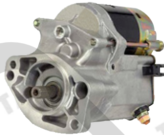
SN-1791 1.0kw,CW
