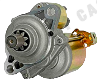
SA-1941 1.0kw,CW,9T,PMGR
